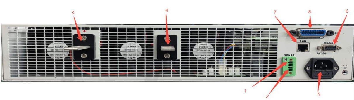
图 3-4 后面板
