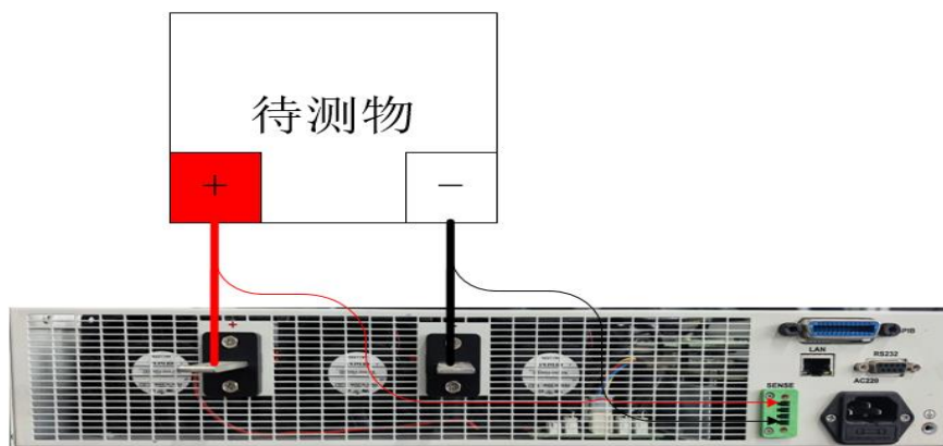
图 4-4 远端电压补偿接线方式
