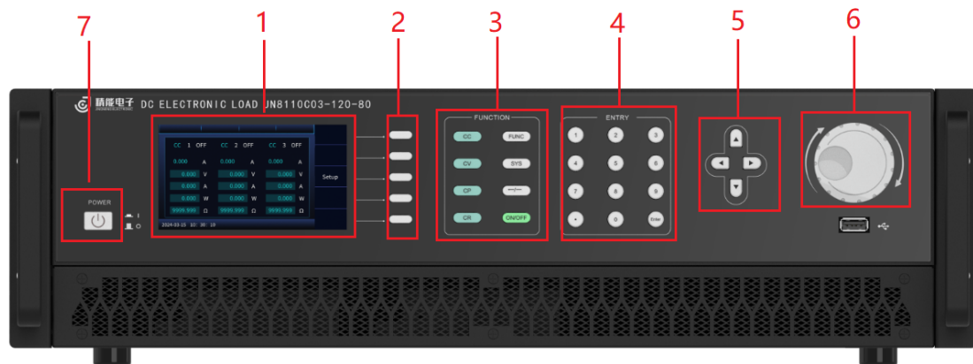
图 3-3 前面板
