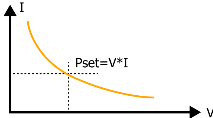
图 5-5 CP 模式
