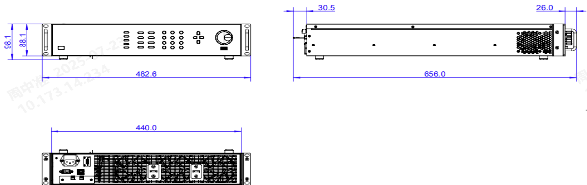
图 3-2 单机尺寸
