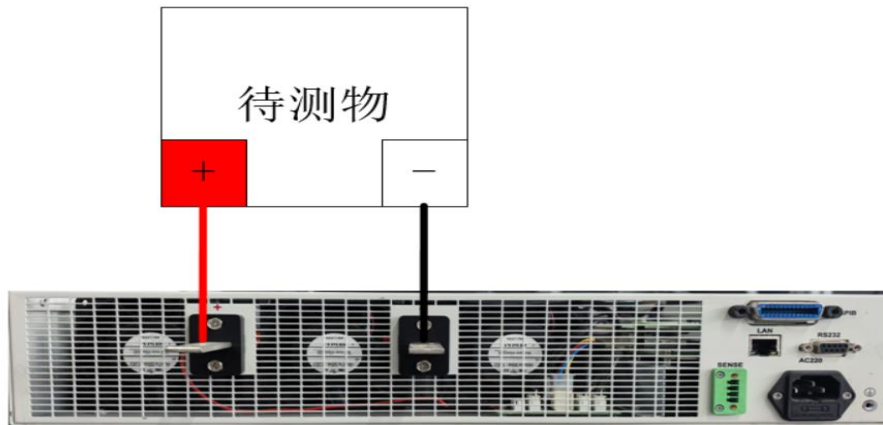
图 4-3 拉载接线方式
